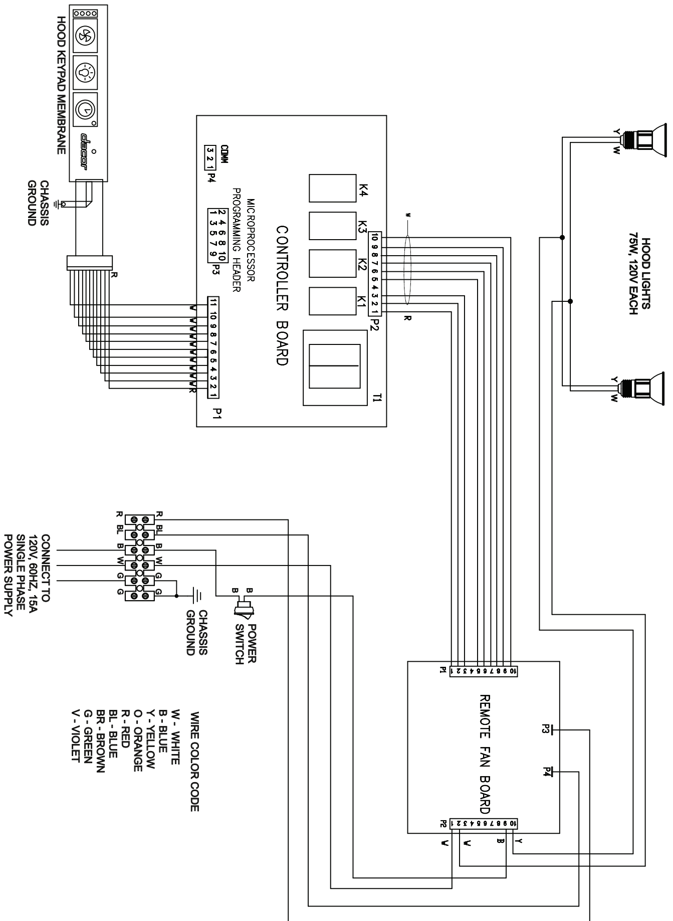
Wiring Diagram: Models EHR30 - EHR36 - EHR42
