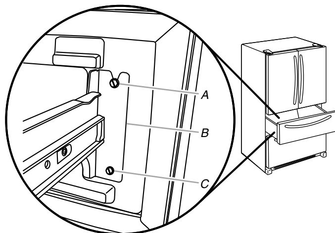
A. Loosen top screws
