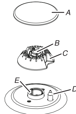
A. Chapeau de brûleur B. Ouverture du tube d'arrivée de gaz C. Base du brûleur D. Électrode d'allumage E. Support du gicleur
