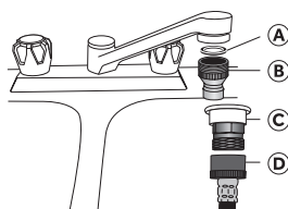
Filetages Internes
